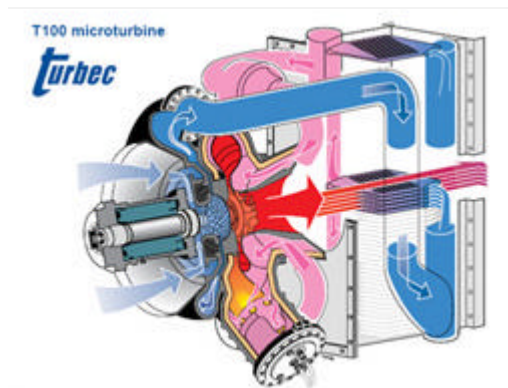
Aufbau einer Turbec-Mikrogasturbine
